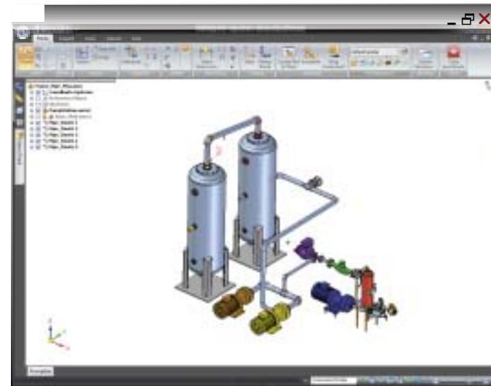
Rys. 10. Niewielkie pochylenie rur w instalacjach ściekowych to jedno z wielu udoskonaleń wprowadzonych do połączeń rurowych.
