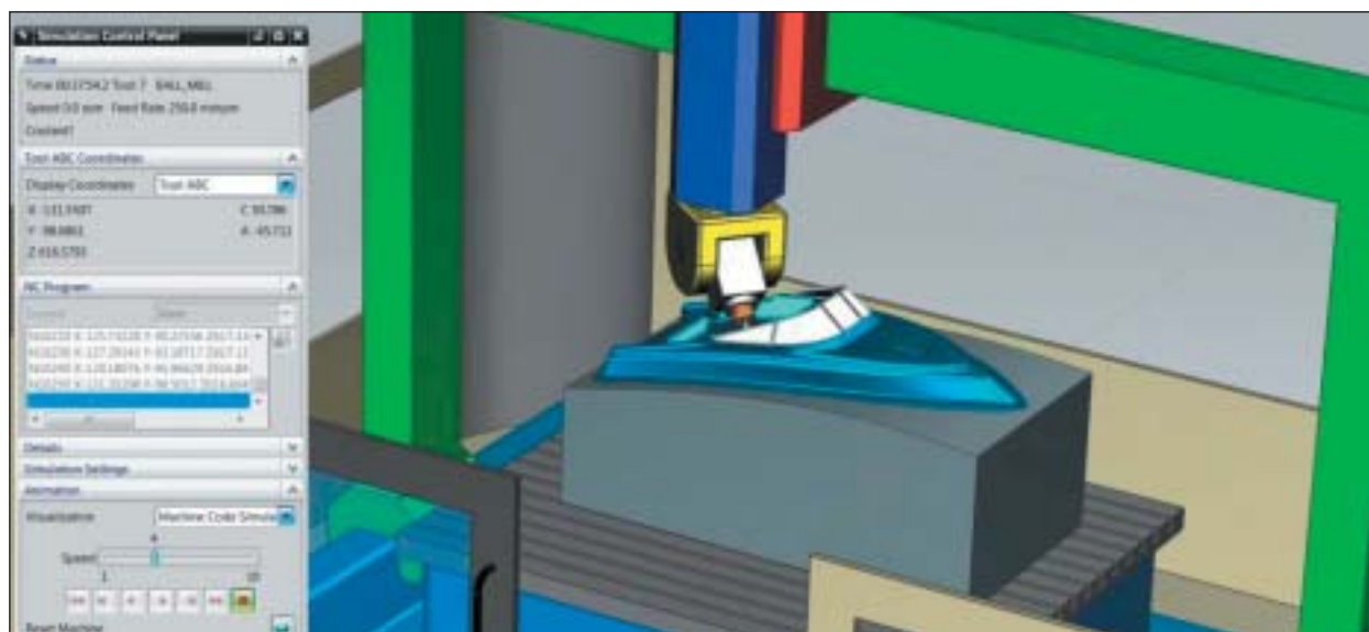
Rys. 2. Symulacja NC w środowisku NX CAM
