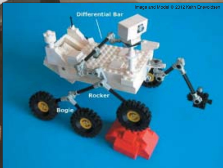
Ten model z klocków Lego, którego autorem jest Keith Enevoldsen, znakomicie demonstruje zasadę działania „drażka różnicowego”...
